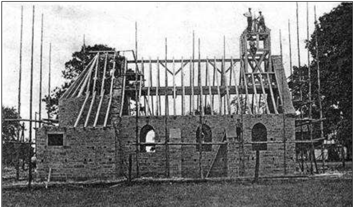
Abbildung 2.2-1 - Ansicht von der Südseite, während der Errichtung des Dachstuhls.
